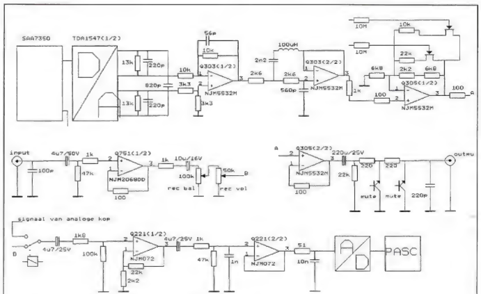
Marantz DD-92
